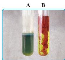
(A) رسوب سبز آهن (II) هیدروکسید (B) رسوب قرمز قهوه‌ای آهن (III) هیدروکسید
